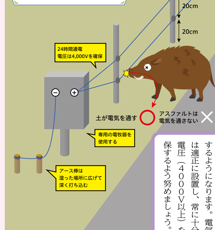
野生動物が感電するしくみ
